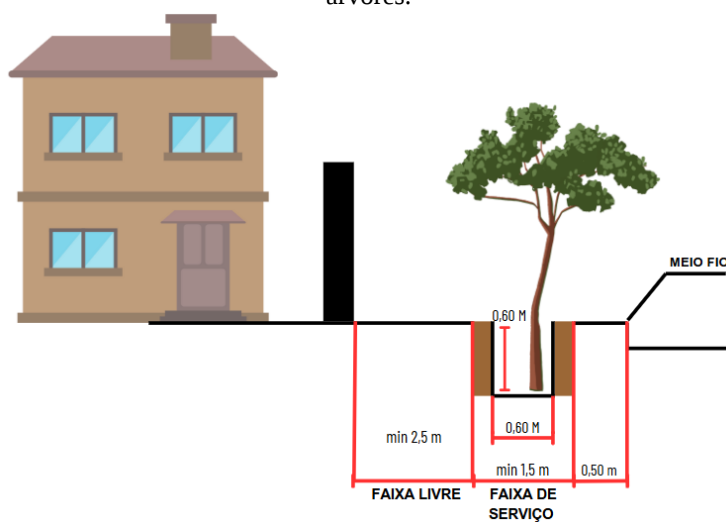
Figura 4. Dimensões mínimas de coveamento e calçamento a serem consideradas no momento do plantio das árvores.
